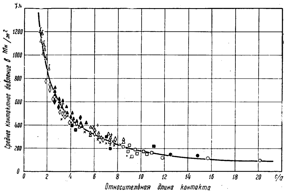
Рис. 1. Зависимость среднего контактного давления от относительной длины контакта при переднем угле \gamma = 10^\circ : \lambda — бронза БрБ2, НВ=320, резец — ВК8; \square — сталь У12, отожженная, резец Т15К6 (по данным нашим и Н. Н. Зорева); \blacktriangle — бронза БрБ2, НВ=200, резец — ВК8; \triangle — бронза БрБ2, НВ=110; резец — ВК8; \times — сталь 12ХНЗ, отожженная, резец Т15К6; \square — медь, резец — Р9; + , \bullet , \circ — опыты Н. Н. Зорева (стали 10, 20, 18ХНВ)
