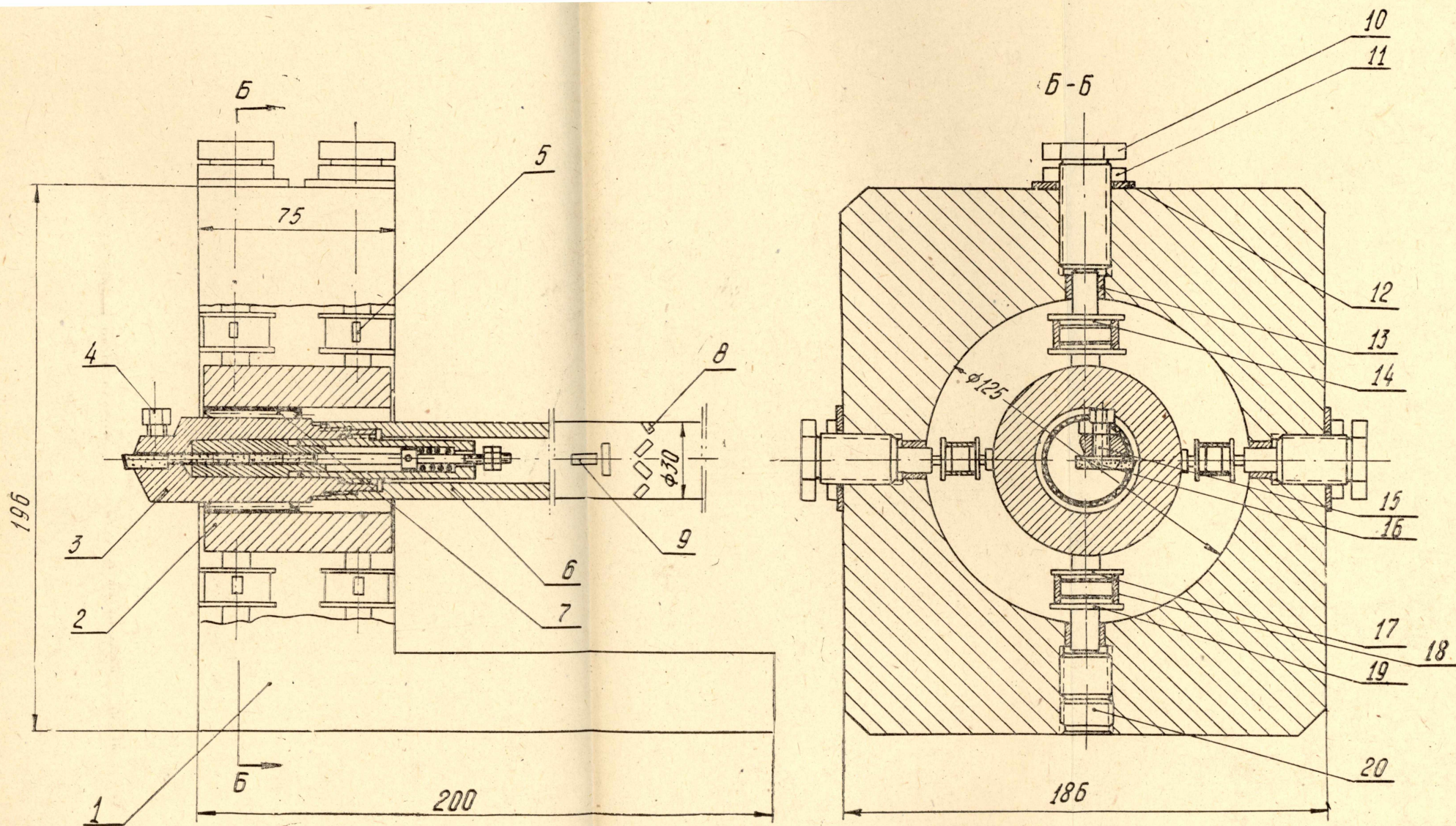
Рис. 2. Динамометрическая установка
