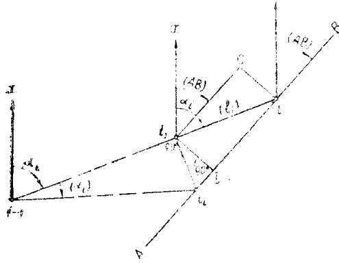
Рис. 2) Схема смещения вершины полигона за счет уравнивания.
