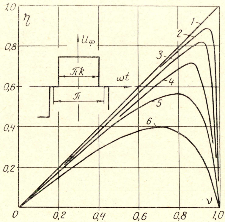
Рис. 1. К. п. д. бесщеточных двигателей. а — при независимом включении обмоток: 1 — идеальный случай; 2 — k=0,75 , \tau_c=1,0 ; 3 — k=0,75 , \tau_0=0,5 ; 4 — k=0,75 , \tau_0=0,2 ; 5 — k=0,75 , \tau_0=0 ; 6 — k=1,0 , \tau_0=0 . б — при соединении фаз «звездой» либо «треугольником»: 1 — идеальный случай; 2 — k = \frac{5}{6} , \tau_0=1,0 ; 3 — k = \frac{5}{6} , \tau_0=0,5 ; 4 — k = \frac{5}{6} , \tau_0=0,2 ,
