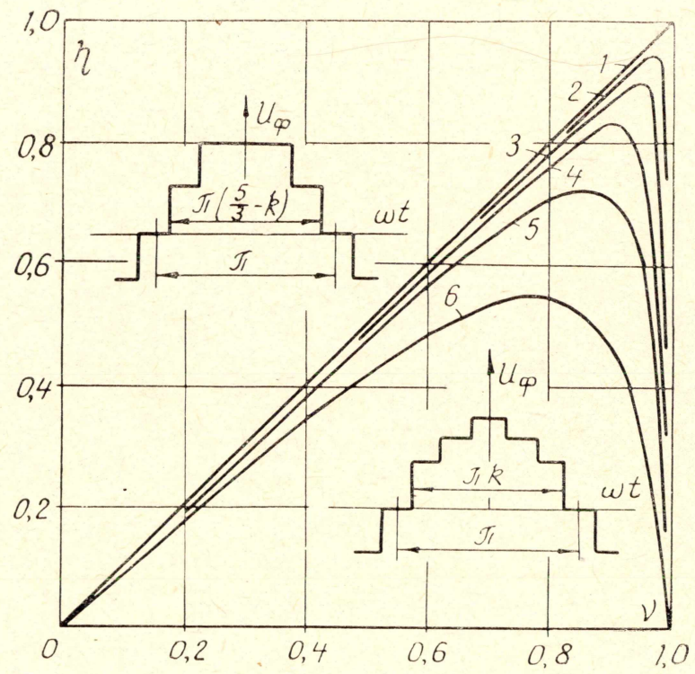
Рис. 1. К. п. д. бесщеточных двигателей. а — при независимом включении обмоток: 1 — идеальный случай; 2 — k=0,75 , \tau_c=1,0 ; 3 — k=0,75 , \tau_0=0,5 ; 4 — k=0,75 , \tau_0=0,2 ; 5 — k=0,75 , \tau_0=0 ; 6 — k=1,0 , \tau_0=0 . б — при соединении фаз «звездой» либо «треугольником»: 1 — идеальный случай; 2 — k = \frac{5}{6} , \tau_0=1,0 ; 3 — k = \frac{5}{6} , \tau_0=0,5 ; 4 — k = \frac{5}{6} , \tau_0=0,2 ,
