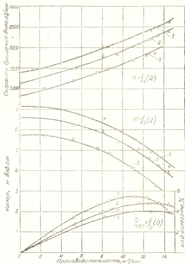
Рис. 2. Характеристика турбонасоса БН-15×4 1 — при давлении 5 атм и расходе воздуха 1,85 м³/мин. 2 — при давлении 4 атм и расходе воздуха 1,56 м³/мин. 3 — при давлении 3 атм и расходе воздуха 1,21 м³/мин.
