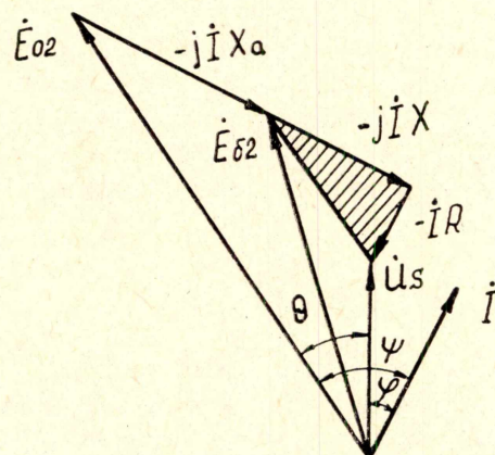
Рис. 2. Векторная диаграмма эдс бесконтактного однофазного генератора
