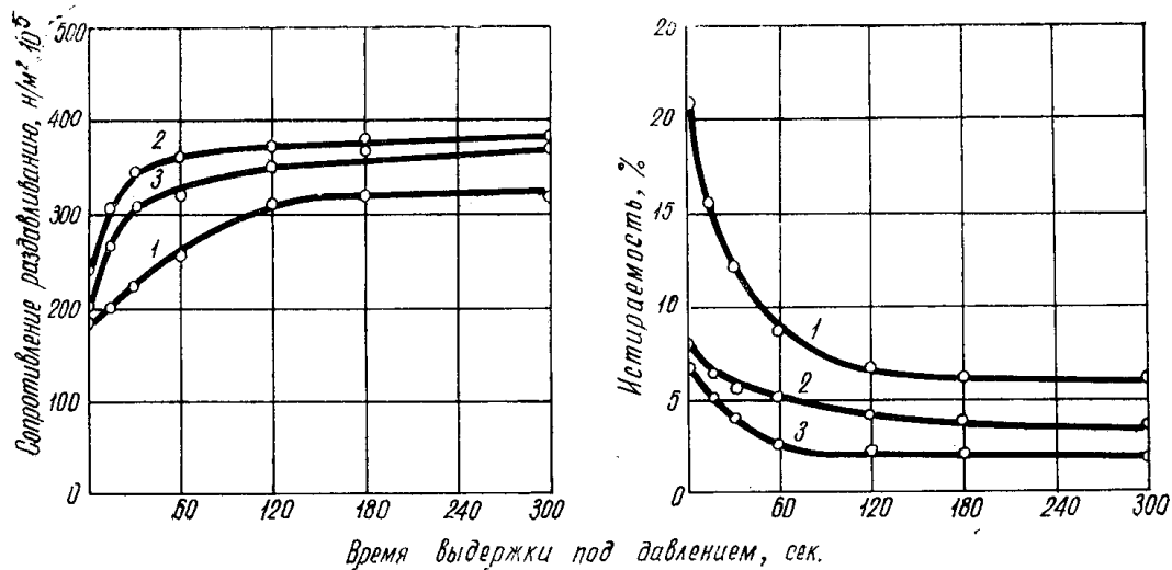
Рис. 2. Влияние времени выдержки под давлением на прочность термобрикетов. 1 — торф со степенью разложения 5%, 2 — 25%, 3 — 55%.
