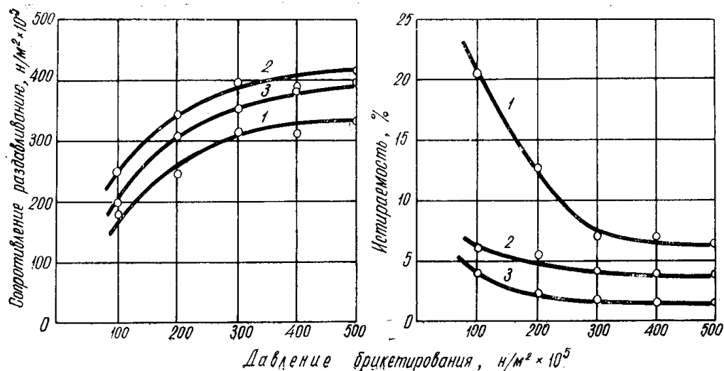
Рис. 1. Влияние давления брикетирования на прочность термобрикетов. 1—торф со степенью разложения 5%, 2 — 25%; 3 — 55%.
