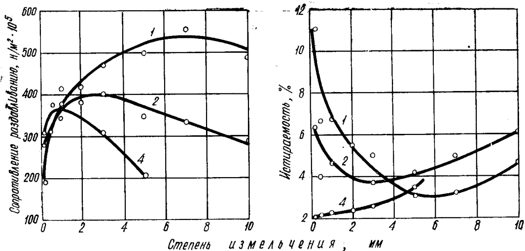
Рис. 3. Влияние крупности частичек торфа на прочность термобрикетов. 1 — торф со степенью разложения 5%, 2 — 25%, 3 — 55%.
