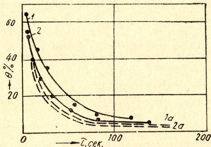
Рис. 1. Зависимость доли ( \Theta %) металла, остающегося в амальгаме, к моменту \tau от величины \tau для амальгам Cd (1) и Zn (2) в растворе 0,5 М K_2SO_4 + 5 \cdot 10^{-4} М MeSO_4 . 1a и 2a — теоретические кривые по (8).
