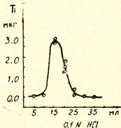
Рис. 2. Кривая элюирования хлоридного комплекса титана.
