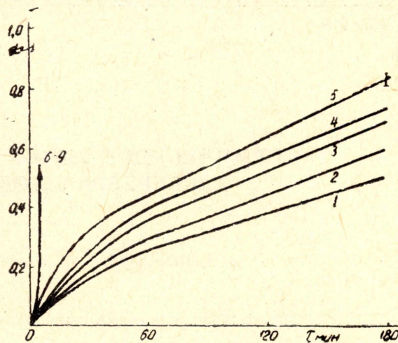
Рис. 1. Термическое разложение азидов серебра при 235°C в вакууме чистого (1) и с добавками: \text{CuO} — 3,3; 4,76 и 9,9 вес % — кривые 2, 3, 4 — соответственно; \text{Cu}_2\text{O} — 3,4 вес % — кривая 5; и \text{AgN}_3 с \text{Cu}_2\text{O} (8%), \text{Cu}_2\text{S} (4÷10%), \text{Cu}_2\text{Se} (10%), \text{CuO} (20%) — кривые 6—9 — вспышка.
