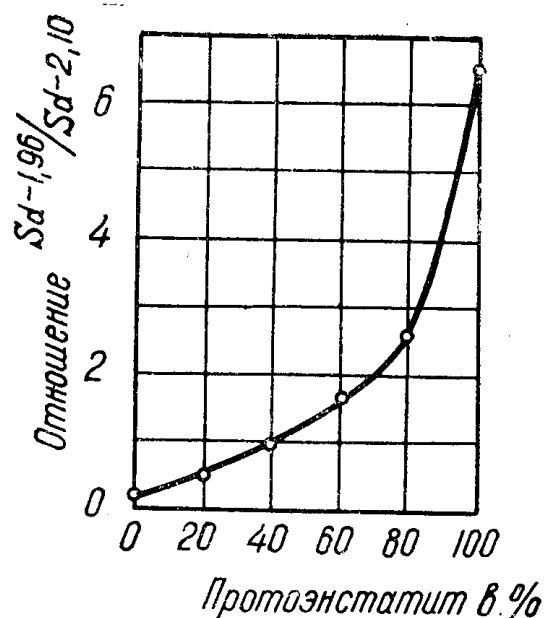
Рис. 1. Зависимость величин отношения площадей рентгеновской дифракции для d=1,96 \text{ Å} и d=2,10 \text{ Å} от количественных соотношений протоэнстатита и клиноэнстатита в пробе
