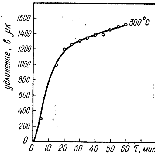
Рис. 2. Расширение образца, обожженного при 300°C, после насыщения водой
