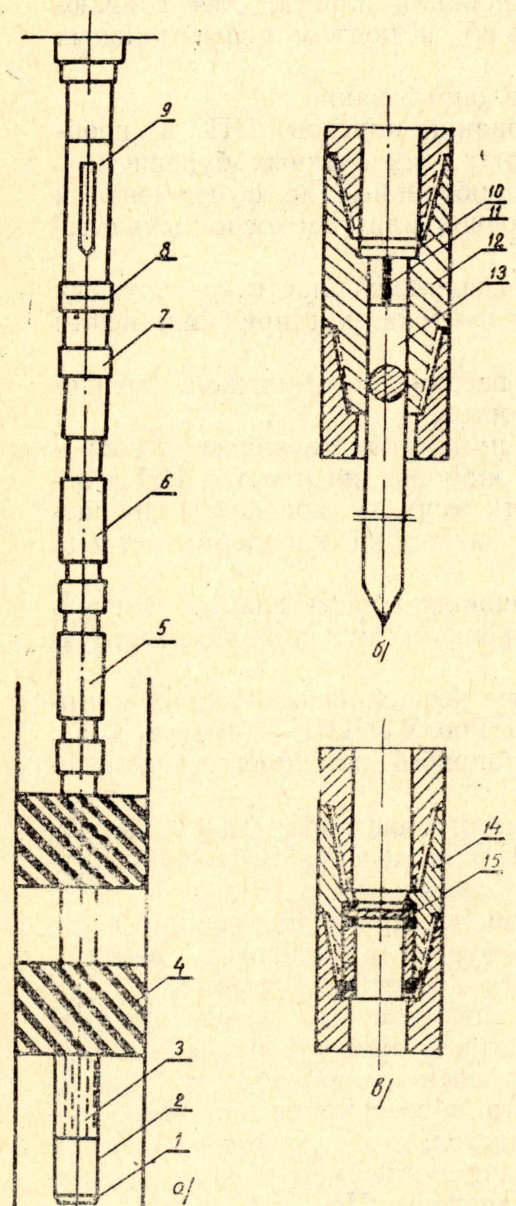
Рис. 1. а — компоновка испытательных инструментов на базе ИП ГрозНИИ; б — устройство подвески штока; в — узел установки чугунной диафрагмы. 1 — башмак, 2 — хвостовик, 3 — фильтр, 4 — спаренный пакер, 5 — уравнильный клапан; 6 — тарельчатый клапан, 7 — стопорное устройство, 8 — чугунная диафрагма, 9 — квадратная штанга, 10 — шпилька; 11 — трос, 12, 14 — переводник, 13 — шток
