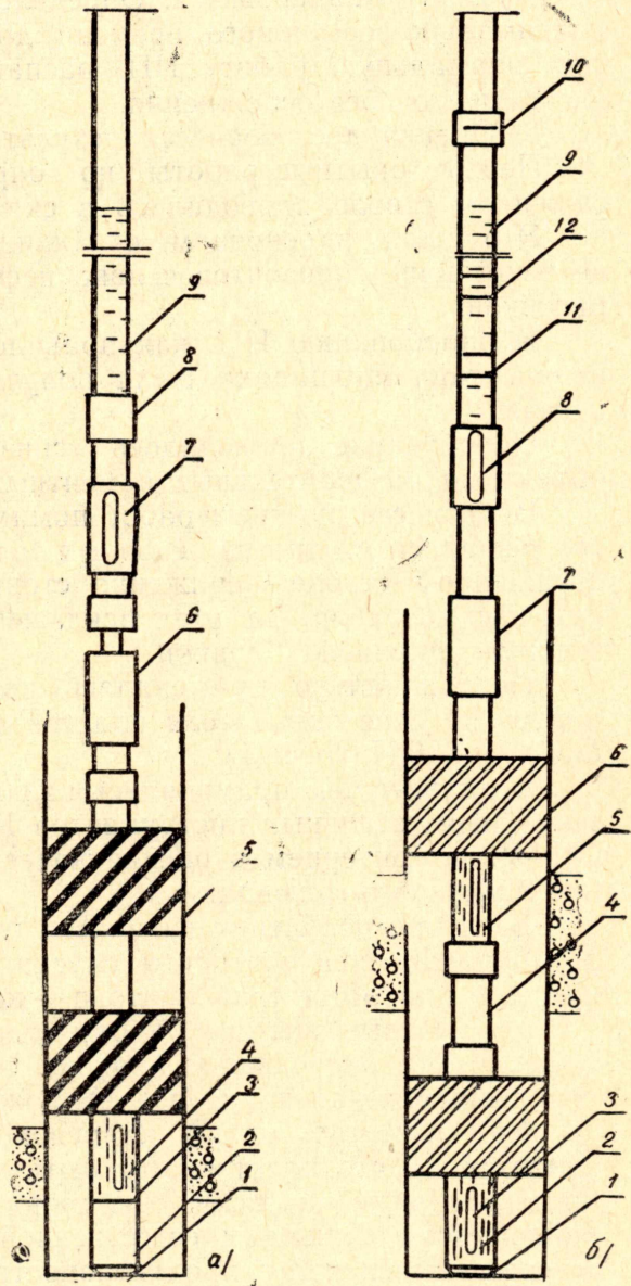
Рис. 2. Компоновка КИИ ГрозУфНИИ: а — со спаренным пакером. 1 — башмак, 2 — хвостовик, 3 — фильтр, 4, 7 — глубинный манометр, 5 — спаренный пакер, 6 — сборка ГрозУфНИИ, 8 — циркуляционный клапан, 9 — бурильные трубы; б — с двойной пакеровкой. 1 — башмак, 2, 5 — фильтр, 3, 8 — глубинный манометр, 4 — уравнильный клапан, 6 — пакер, 7 — сборка КИИ ГрозУфНИИ, 9 — глинистый раствор, 10 — чугунная диафрагма, 11 — бурильные трубы, 12 — стопорное устройство
