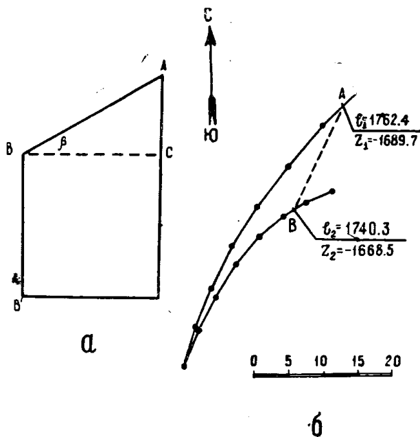
Рис. 1. Определение угла наклона плоскости напластования в керне (а) и направления наклона прямой косоугольного сечения (б)
