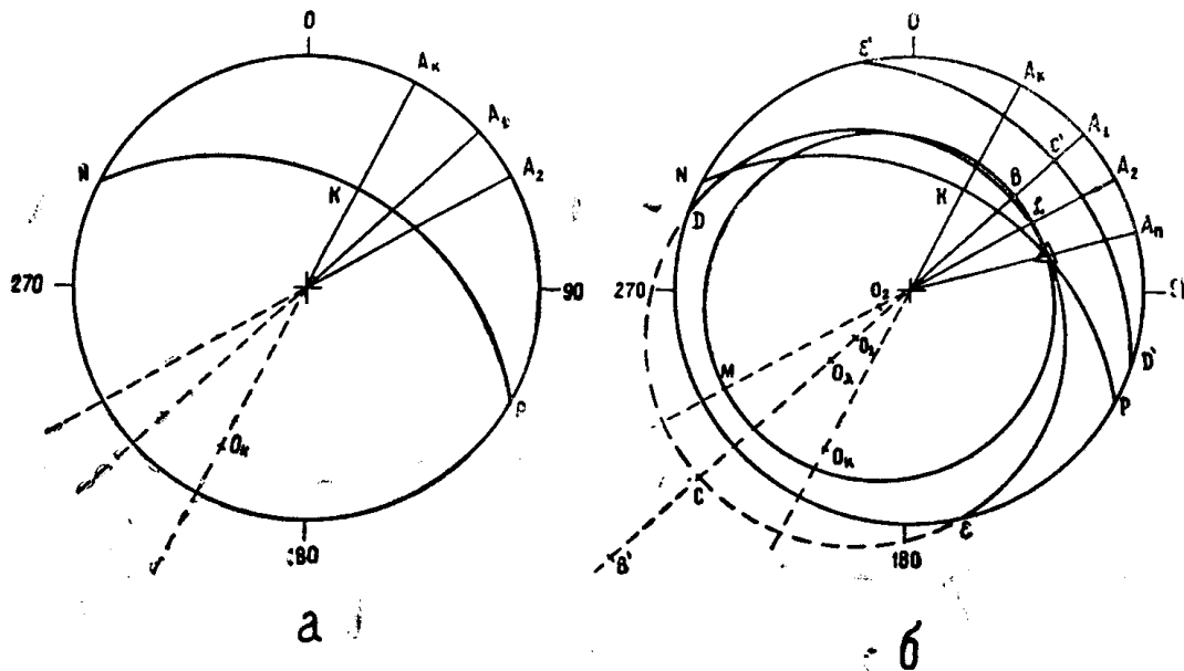
Рис. 2. Определение элементов залегания пласта по прямой косога сечения и двум неориентированным кернам графо-аналитическим методом на стереографической проекции уменьшено вдвое
