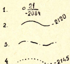
Рис. 1. Структурная карта по кровле пласта Б-Х Мыльджинского месторождения. 1 — пробуренные скважины, числитель — номер скважины, знаменатель — абсолютная отметка кровли пласта Б-Х; 2 — изогипсы кровли пласта Б-Х, 3 — литологическая граница пласта Б-Х, 4 — газо-водяной контакт (условный)
