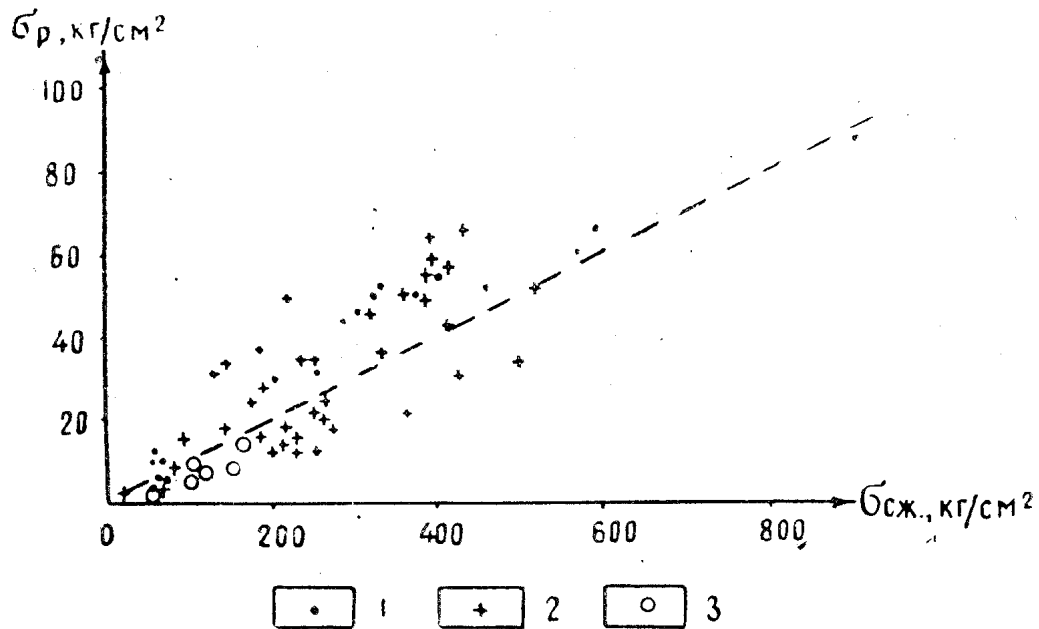
Рис. 1. Зависимость между временным сопротивлением сжатию и разрыву пород Урупского месторождения: 1 — песчаники юры, 2 — песчаники перми, 3 — алевролиты перми
