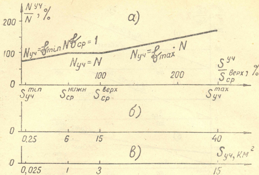
Рис. 2. Характер поведения общей оптимальной кривой функции N_{уч.} = f: N (а) с примерными частными шкалами изменения площадей мелких, средних и крупных участков для пластовых рудных (в) и каменноугольных (б) месторождений
