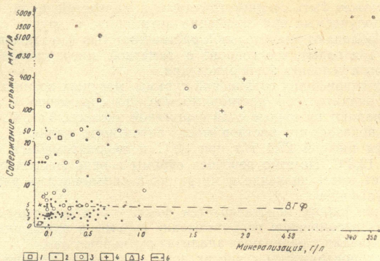
Рис. 1. Распространение сурьмы в природных водах. 1 — поверхностные воды, 2 — грунтовые воды, 3 — рудничные воды, 4 — воды гидротерм, 5 — соленые воды, 6 — верхняя граница фона (вгф)
