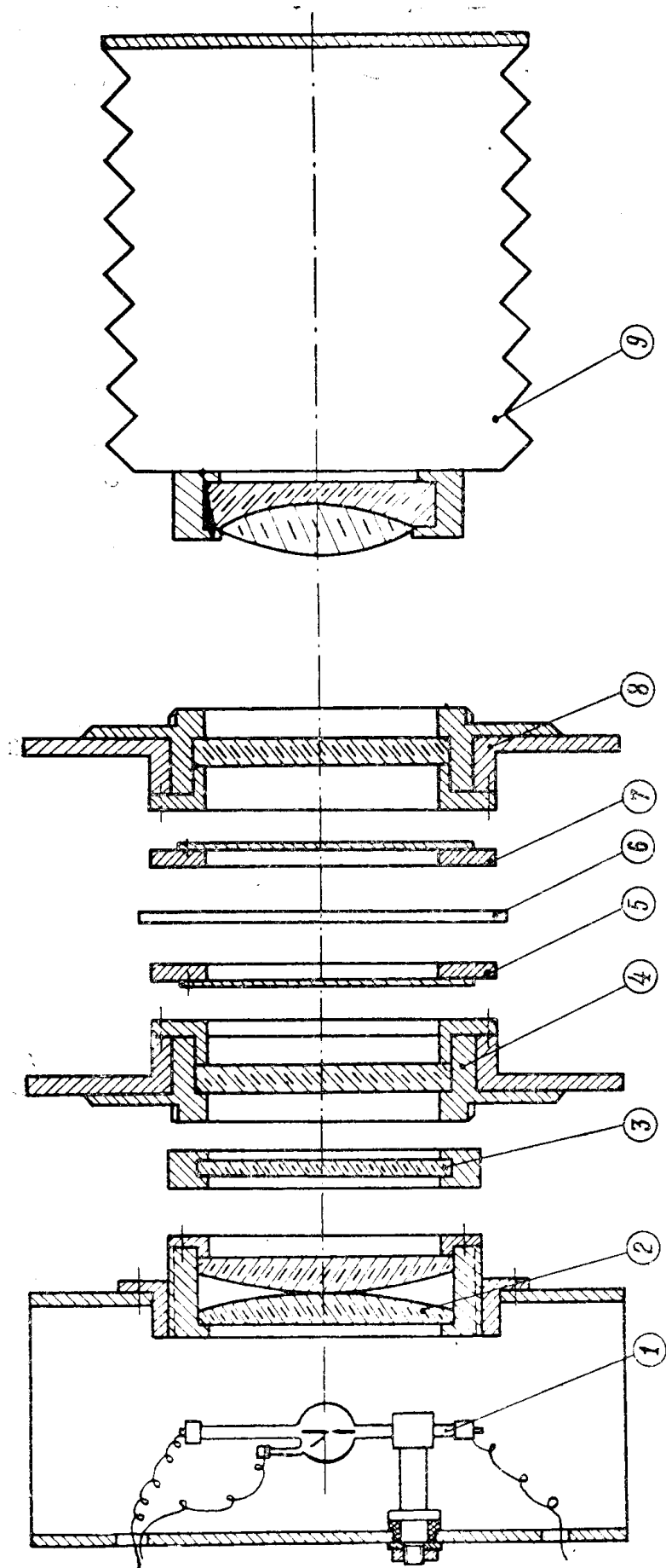
Рис. 1. Оптическая система установки.
