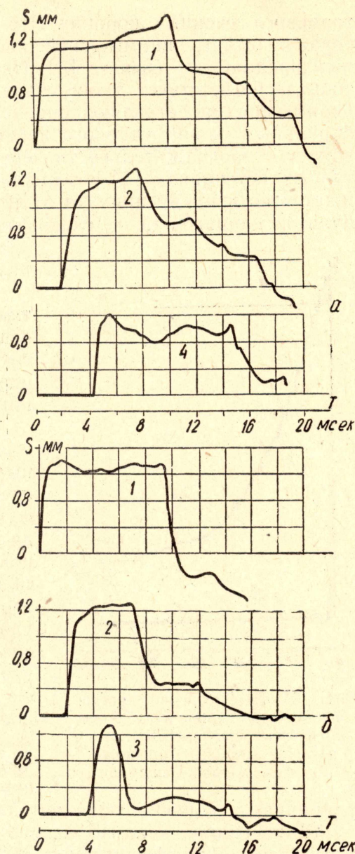
Рис. 2. Перемещение поперечных сечений, фиксированных по длине штанги на расстоянии от ударника: 1 — 0,5 м; 2 — 10,5 м; 3 — 20,5 м; 4 — 25 м; общая длина штанги — 25,5 м
