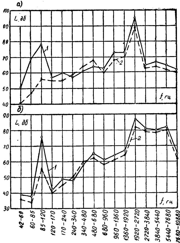
Рис. 1. Спектры вибраций: а) ЭМУ-12 ( n=5400 об/мин), б) ЭМУ-5 ( n=6000 об/мин). 1 — после уравнивания на типовом балансировочном оборудовании; 2 — после уравнивания на Б-1 и Б-2
