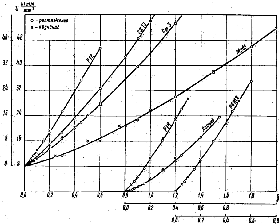
Рис. 1. Кривые течения. По опытам авторов
