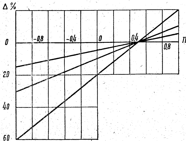
Рис. 3. Отклонения от простого нагружения в случае расчета программы по условным напряжениям при e_i = 5, 10, 20\%
