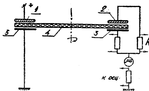
Рис. 1. Схема осциллографирования токов: 1, 2 — индукторы возбуждения и разрядный; 3, 5 — щетки разрядная и зарядная; 4 — ротор
