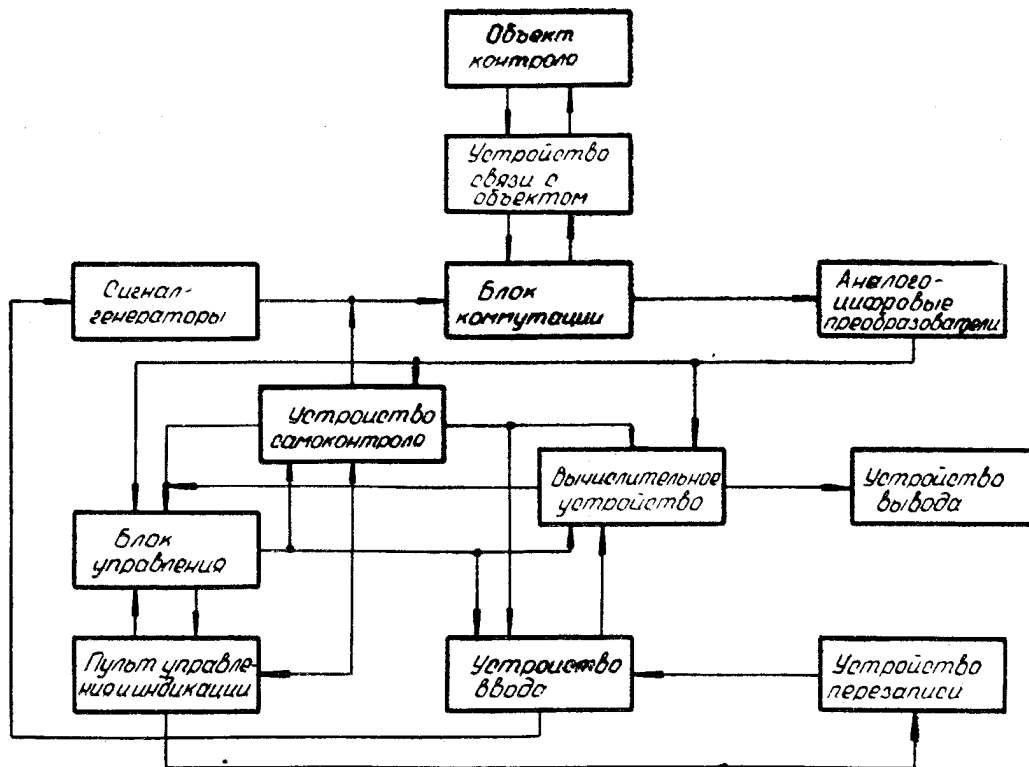
Рис. 1. Блок-схема универсальной САК
