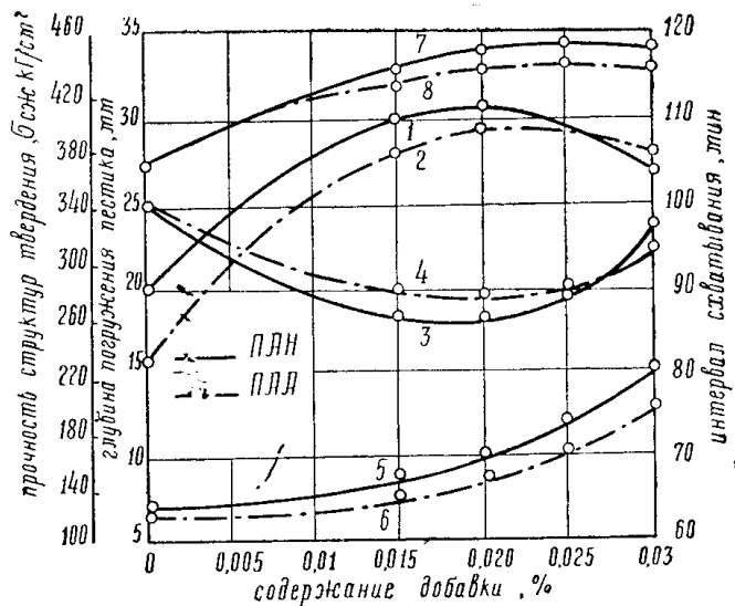
Рис. 1. Структурно-механические свойства цемента.
