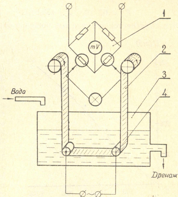
Рис. 1. Схема устройства для измерения общей жесткости воды
