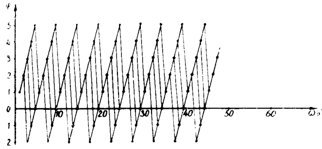
Рис. 3. Распределение фаз в спектре выходного тока смесителя при \frac{\omega_1}{\omega_2} = \frac{5}{6} .
