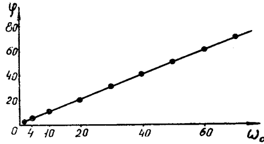
Рис. 1. Распределение фаз в спектре выходного тока смесителя
