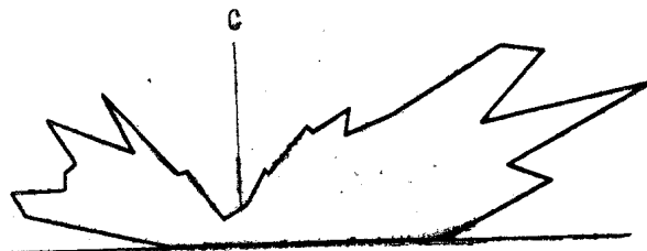
Рис. 4. Роза направленности изодинам \Delta Z .
