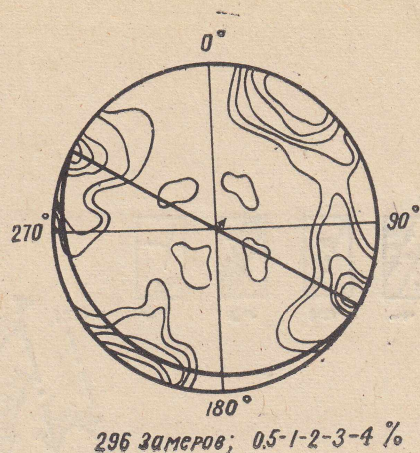
Рис. 2. Характер трещиноватости угольных пластов. Диаграмма элементов залегания трещиноватости, изученной в забое лавы № 7 пл. Поджуринского-1 на шахте «Журинка-3».
