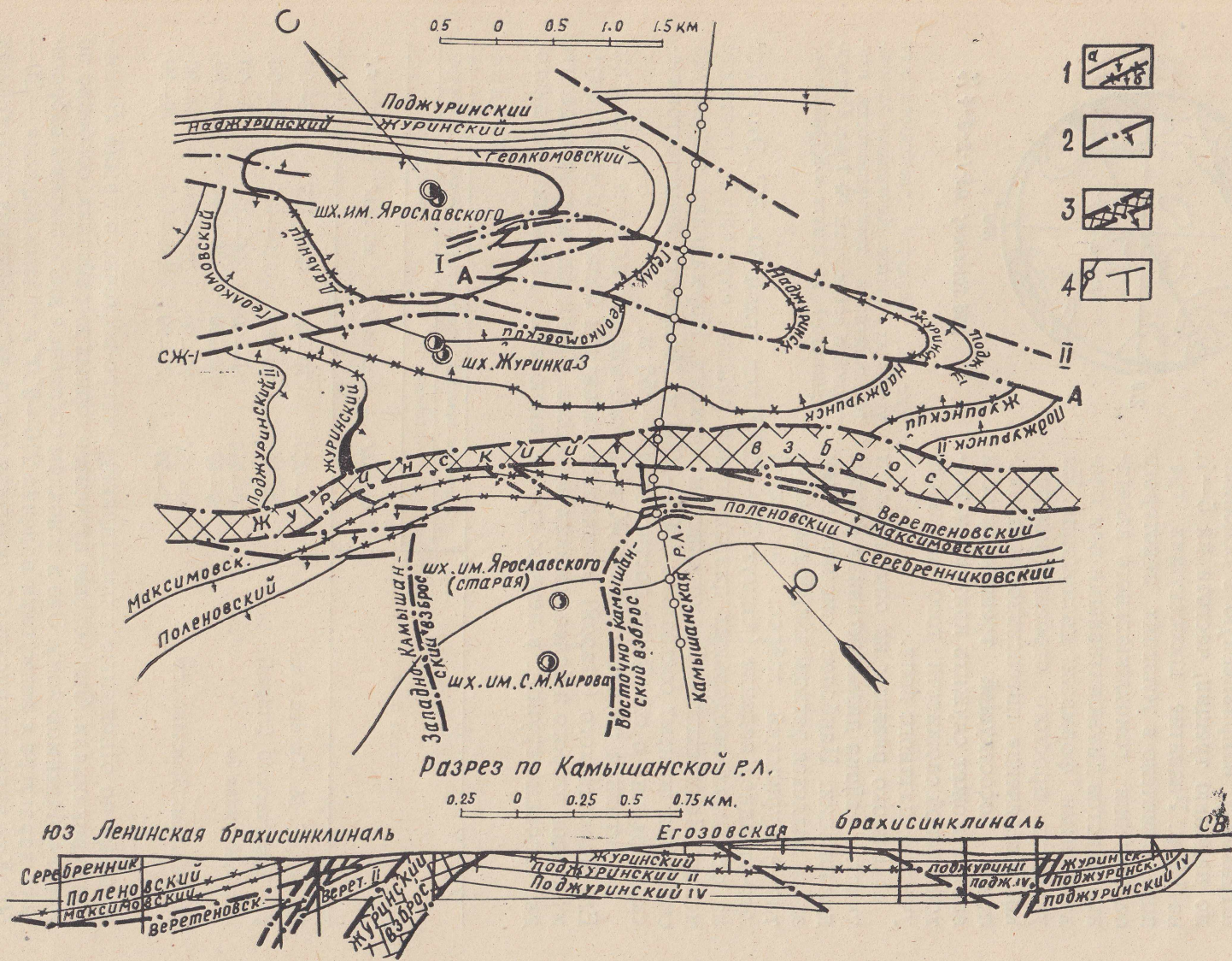
Рис. 1. Характер тектоники северо-восточных шахтных полей Ленинского района. А. Схематический план выходов угольных пластов под наносы. Б. Разрез по Камышанской разведочной линии. 1 — выходы под наносы угольных пластов, а) разведанных; б) отработанных; 2 — дизъюнктивы; 3 — зоны тектонических брекчий в боках дизъюнктивов; 4 — разведочные скважины
