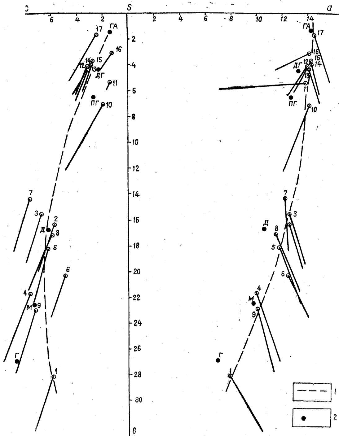
Рис. 1. Диаграмма химического состава пород тыгертышского интрузивного комплекса (по А. Н. Заварицкому). 1 — вариационная линия тыгертышского интрузивного комплекса; 2 — фигуративные точки средних типов по р. Дели (г — габбро, м — мелафир, д — диорит, пг — послекембрийский гранит, дг — докембрийский гранит, га — гранитовый аплит).
