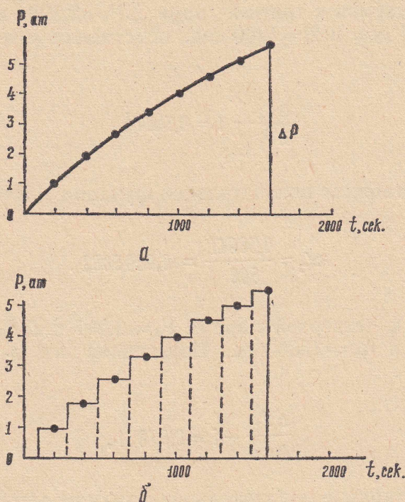
Рис. 1. Площади, отвечающие интегралу Дюамеля:
