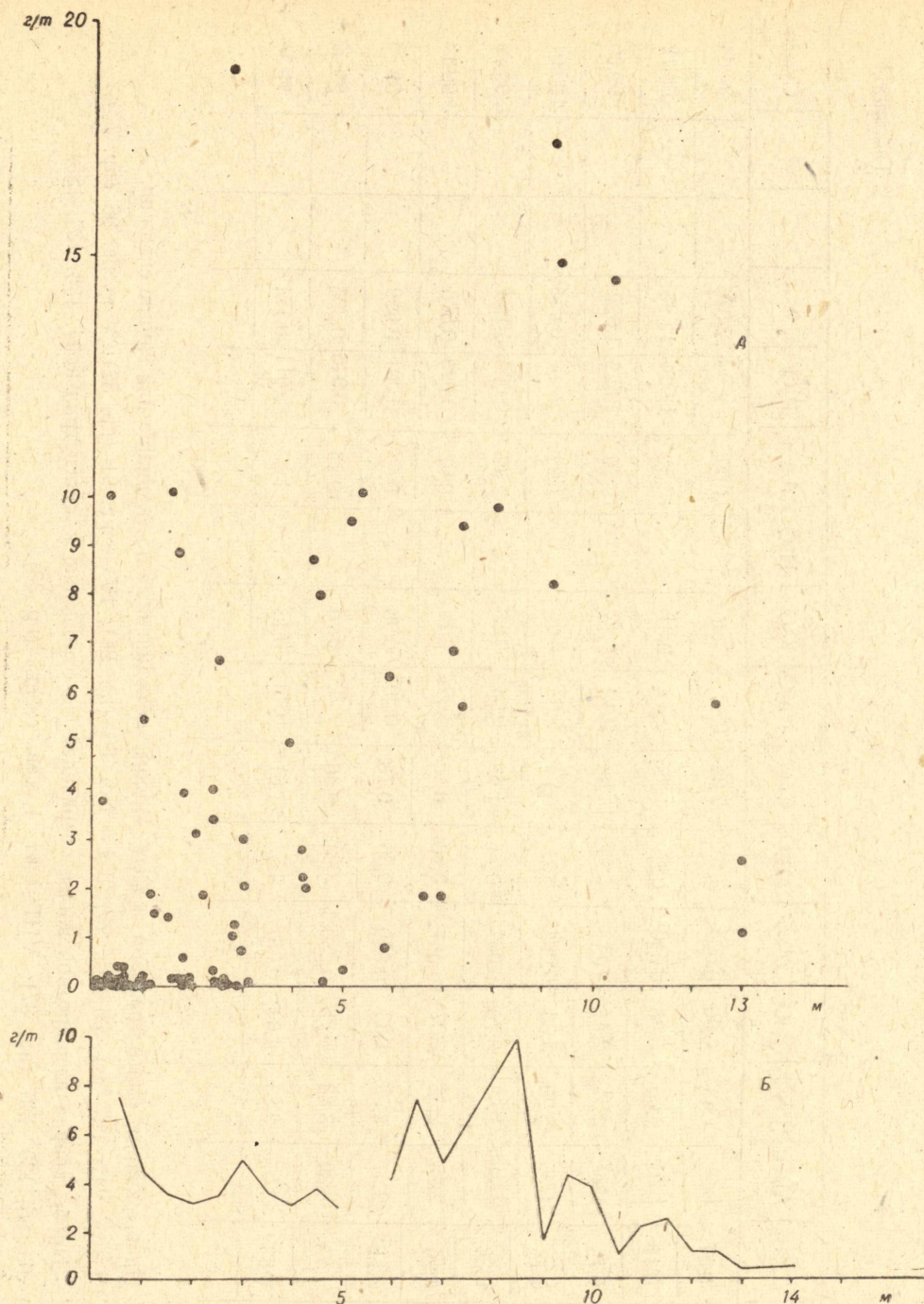
Фиг. 6. а — зависимость содержания Au от суммарной мощности рудных тел (по данным опробования керна колонковых скважин Николаевского месторождения). б — изменение содержания Au в зависимости от расстояния пробы от лежащего бока Магистральной «жилы» (М-ние Николаевское, по данным опробования керна колонковых скважин, осредненные данные по 265 пробам)
