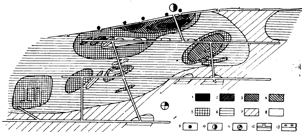
Рис. 1. Схема продольной вертикальной проекции жилы Второй месторождения Талалах
