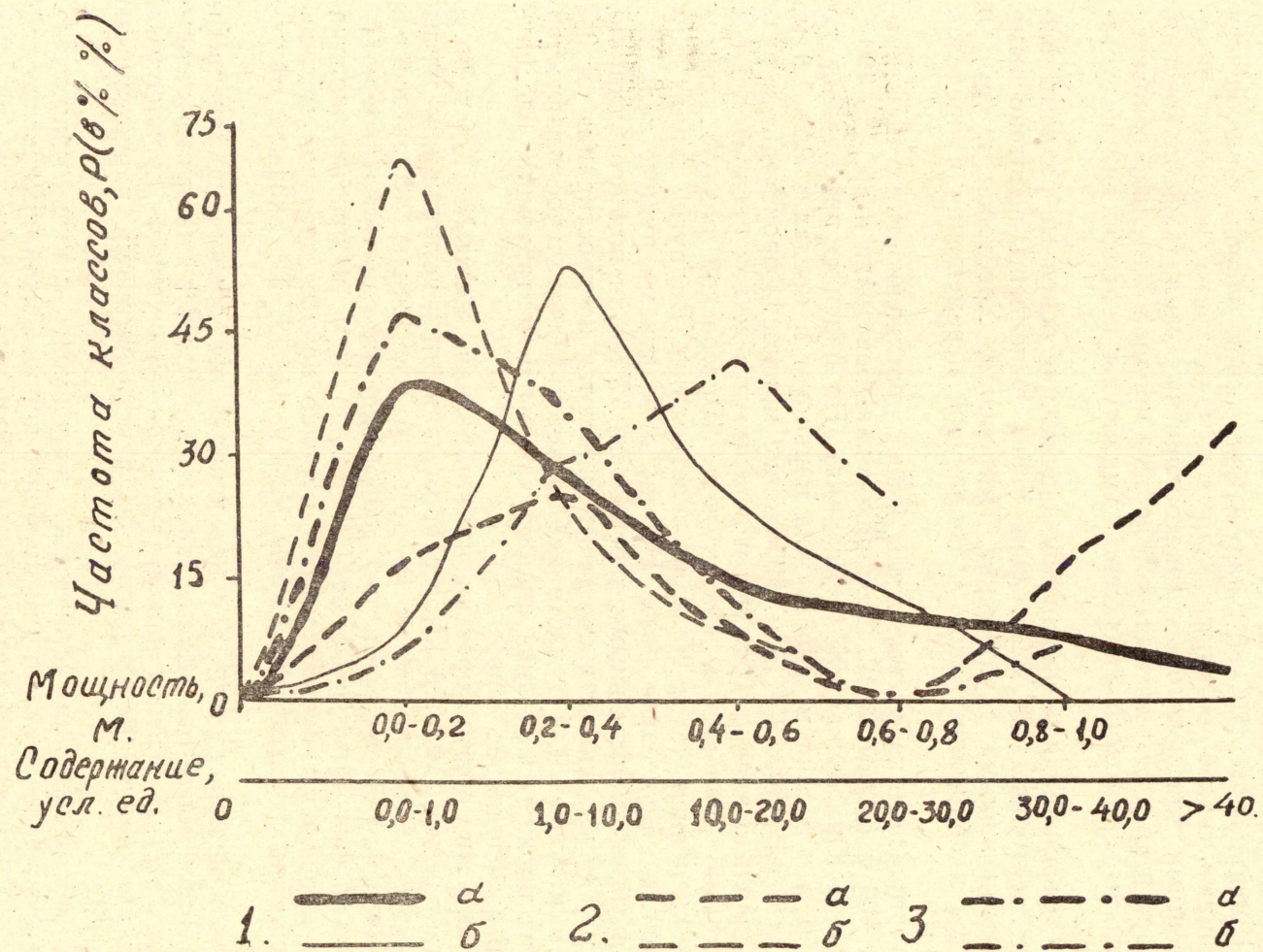
Рис. 1. Диаграмма зависимости содержаний золота (а) и мощности (б) по жиле Верхней от литологического состава вмещающих пород: 1) в гранатово-пироксеновых парагнейсах; 2) в известняках; 3) в амфиболитах
