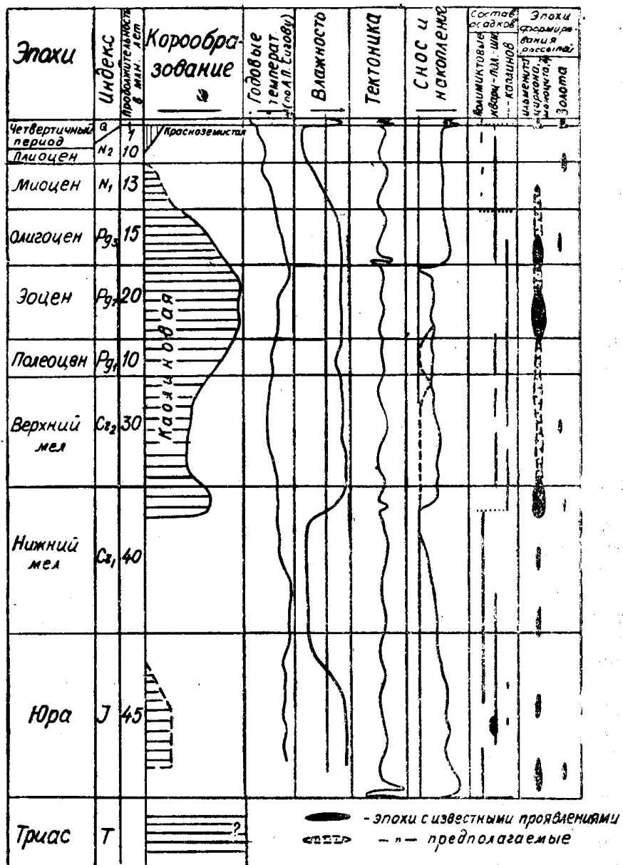
Рис. 1. Схема россыпеобразования на юге Западной Сибири
