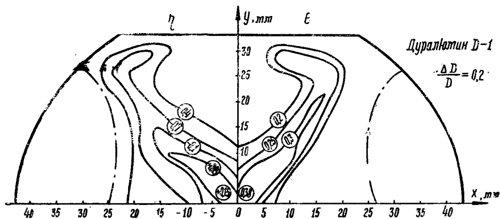
Рис. 2. Изолинии \eta и \epsilon_i для диска из дюралюмина, осаживаемого на 20%
