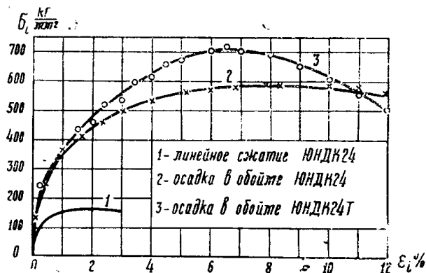
Рис. 1. Кривые деформирования сплавов ЮНДК24 и ЮНДК24Т при одноосном и всестороннем сжатии
