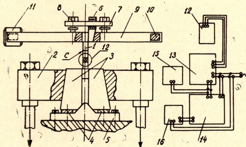
Рис. 1. Схема установки
