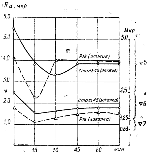
Рис. 1. Изменение чистоты поверхности в зависимости от времени виброобработки
