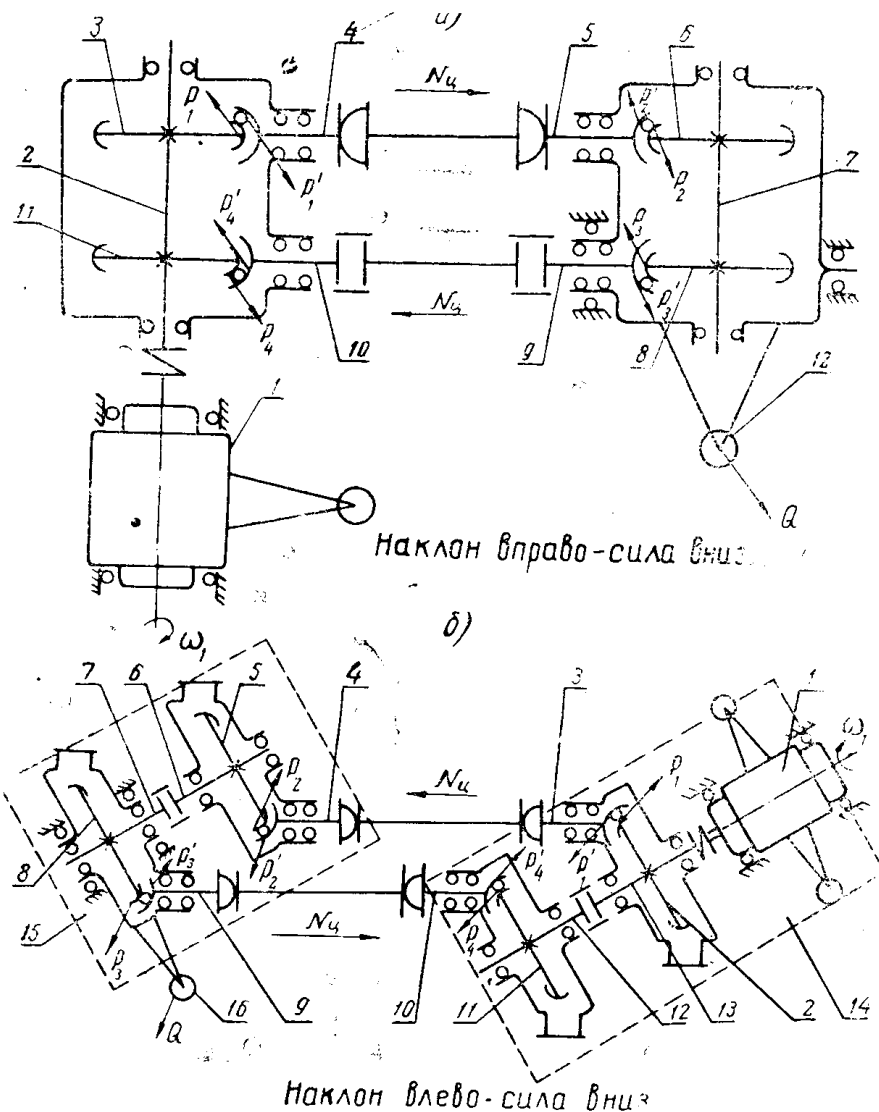
Рис. 1. Схемы установок для испытания передач с пересекающимися осями: а) — при угле пересечения осей \phi = 90^\circ , б) — при угле пересечения осей \phi = 30^\circ и 60^\circ
