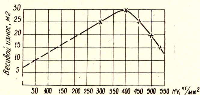
Рис. 2. Зависимость изнашиваемости электронаплавов свободным абразивным зерном от твердости
