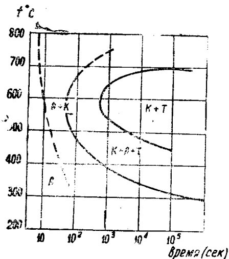
Рис. 3. Диаграмма изотермического распада аустенита высокомарганцовистой стали Г13
