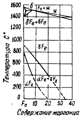
Рис. 1. Диаграмма состояния железо — марганец
