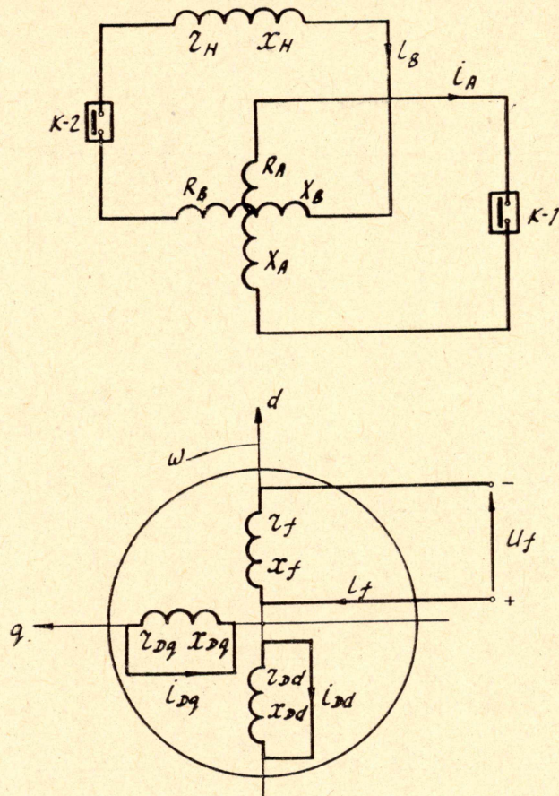
Рис. 1. Принципиальная схема электромашиного источника импульсов.
