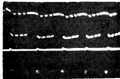
Рис. 7. Клиппированная речь и выходной сигнал интонометра
