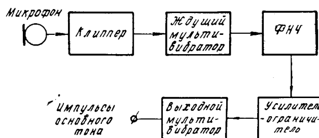
Рис. 1. Блок-схема интонометра
