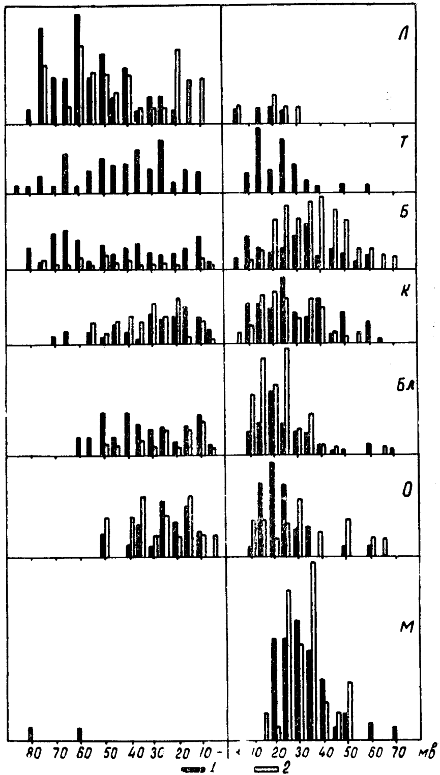
Рис. 1. Гистограмма тэс пиритов (месторождения: Л — Любавинское, Т — Гарданское, К — Коммунарское, Бла — Балахчинское, О — Ольховское, М — Многовершинное), 1 — из кварцевых жил; 2 — из окolorудно измененных пород
