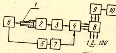
Рис. 2. Блок-схема устройства автоматического учета литых чугунных труб
