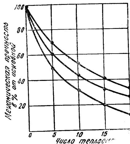
Рис. 2. Зависимость \sigma_{сж} от числа тепловых циклов: верхняя кривая — образцы на сыром тремолите; средняя кривая — образцы на синтезированном диоксиде; нижняя кривая — образцы стеатитовой керамики П-5
