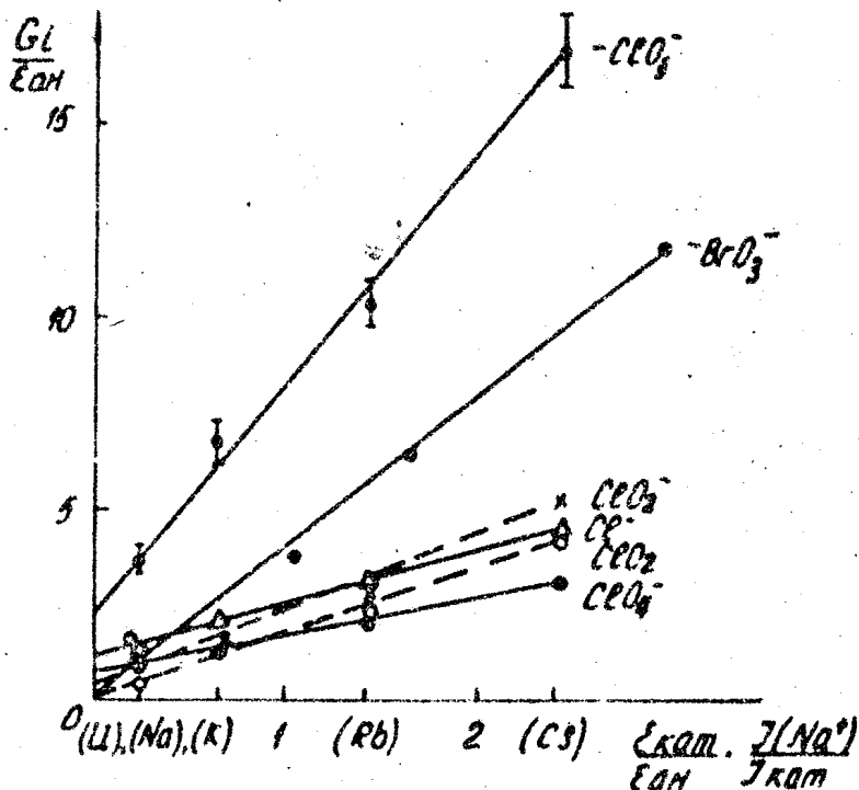
Рис. I. Зависимость выхода продуктов радиолитиза облученных хлоратов и броматов от электронных доз аниона и катиона.
