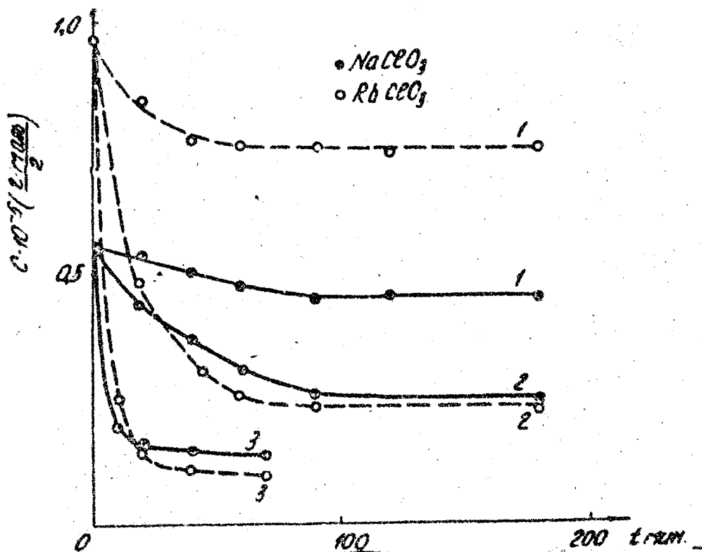
Рис. 3. Изменение концентрации двуокиси хлора в хлоратах при прогреве. 1 - 100^\circ C ; 2 - 130^\circ C ; 3 - 150^\circ C
