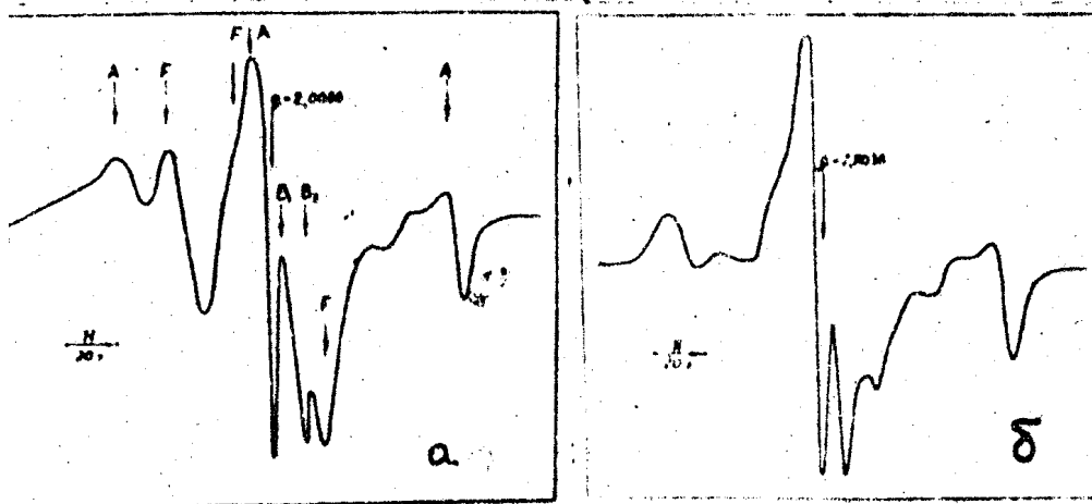
Рис. 2. Спектры ЭПР \gamma -облученных микрокристаллов \text{AgBr} .
