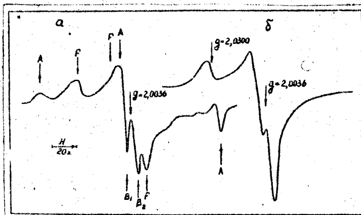
Рис. 4. Спектры ЭПР \gamma -облученных в вакууме микрокристаллов \text{AgBr} . Доза
