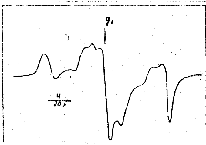
Рис. 3. Спектр ЭПР \gamma -облученных при -196^{\circ}\text{C} микрокристаллов \text{AgBr} . Доза облучения 1 Мрад. Температура регистрации спектра -120^{\circ}\text{C} .
