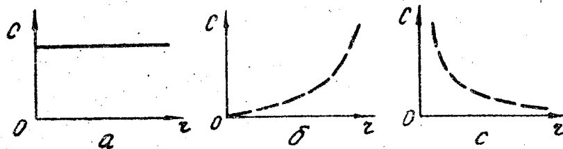
Рис. I. Распределение примесей по объему кристаллов
